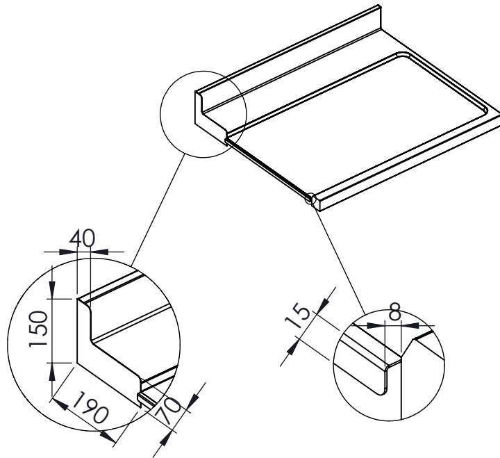
DETTAGLIO SCALA 1 : 2
